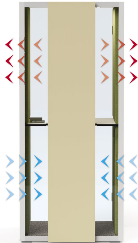
Rückwand aus Glas mit vertikaler Lüftungseinheit, Akustikissen seitlich oberhalb Tischablage. Frischluftzufuhr und Abluft seitlich über die Lüftungseinheit aussen, Luftumwälzung ca. 150m 3 /Std.. Breite 100 cm, Tiefe 100 cm, Höhe 225 cm.
